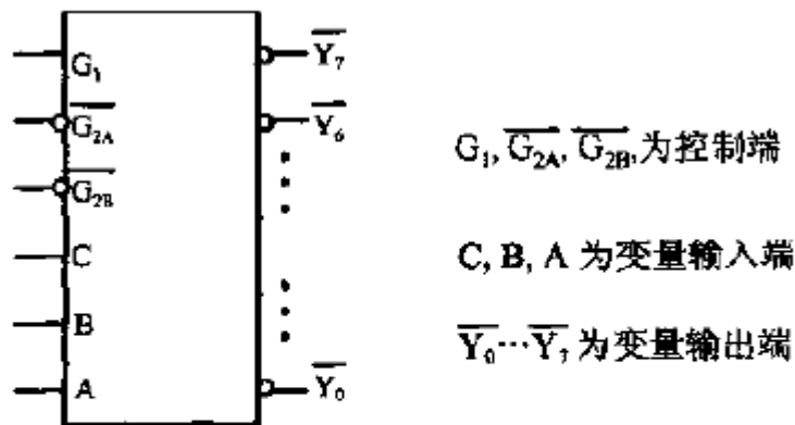
74 138 译码器
