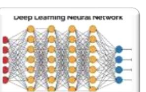
深度学习
