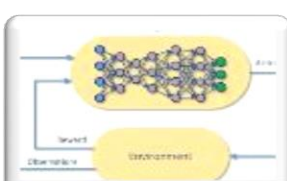
强化学习
