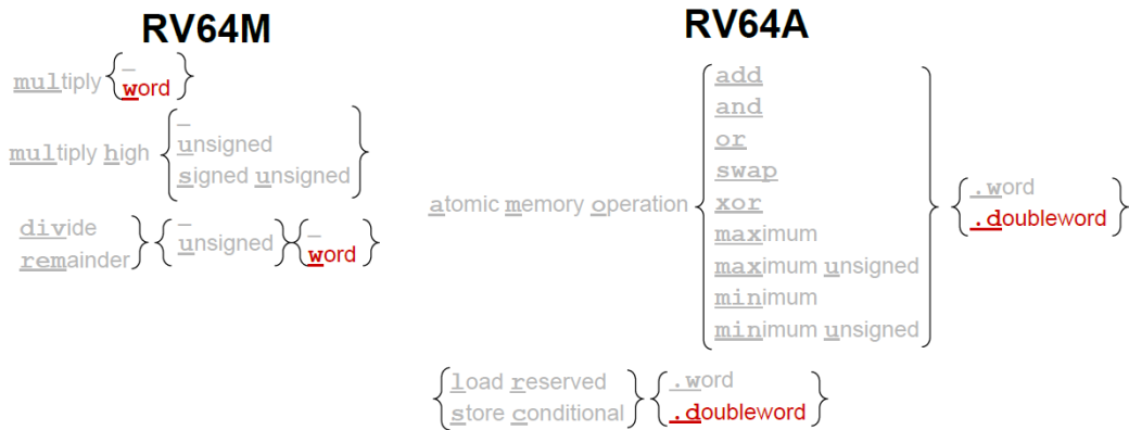
图 9.2: RV64M 和 RV64A 指令图示
