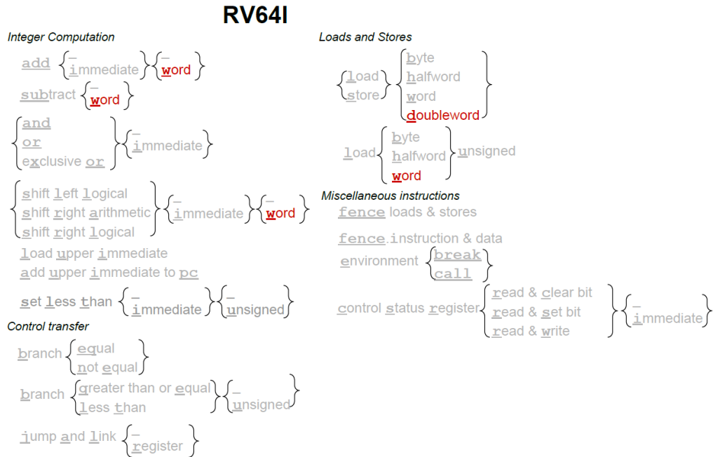
图 9.1: RV64I 指令图示。带下划线的字母从左到右连起来构成 RV64I 指令。灰色部分是扩展到 64 位寄存器的旧 RV64I 指令，而暗（红色）部分是 RV64I 的新指令。
