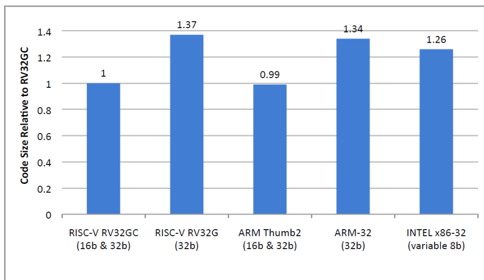
图1.5: RV32G, ARM-32, x86-32, RV32C和Thumb-2程序的相对大小。最后两个ISA是以短代码长度为目标的。这些程序是使用GCC编译器的SPEC CPU2006基准测试。与RV32C相比，Thumb-2的代码短小的优势是由于在进入程序时Load and Store Multiple的节省。RV32C没有包含它们，以保持与RV32G指令的一对一映射，RV32G省略了Load and Store Multiple以降低高端处理器的实现复杂性（见下文）。第七章介绍了RV32C。RV32G表示RISC-V扩展（RV32M，RV32F，RV32D和RV32A）的流行组合，正确称为RV32IMAFD。[Waterman 2016]
